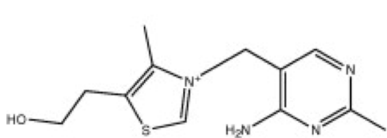
Thiamin, B1
