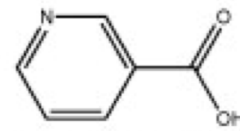
Niacin, B3
