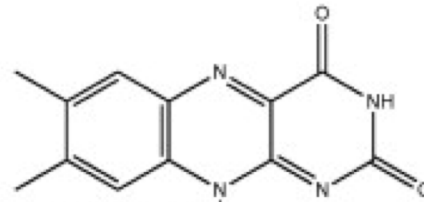
Riboflavin, B2
